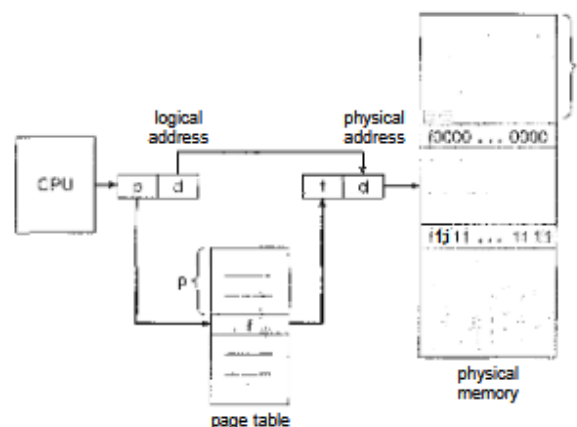
Figure 12.1 Paging hardware.
